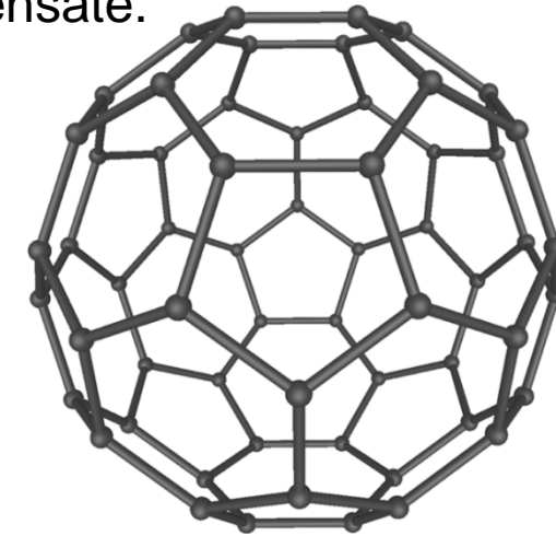
C 60
